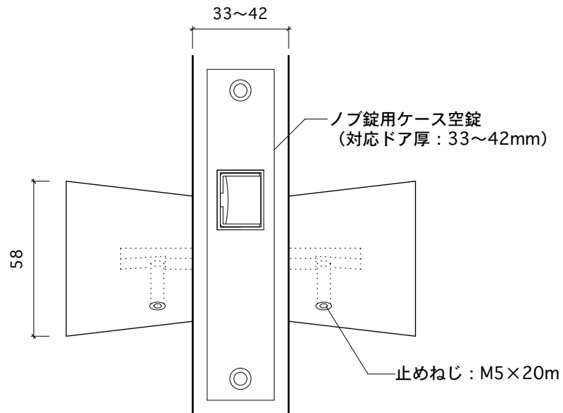
側面図
