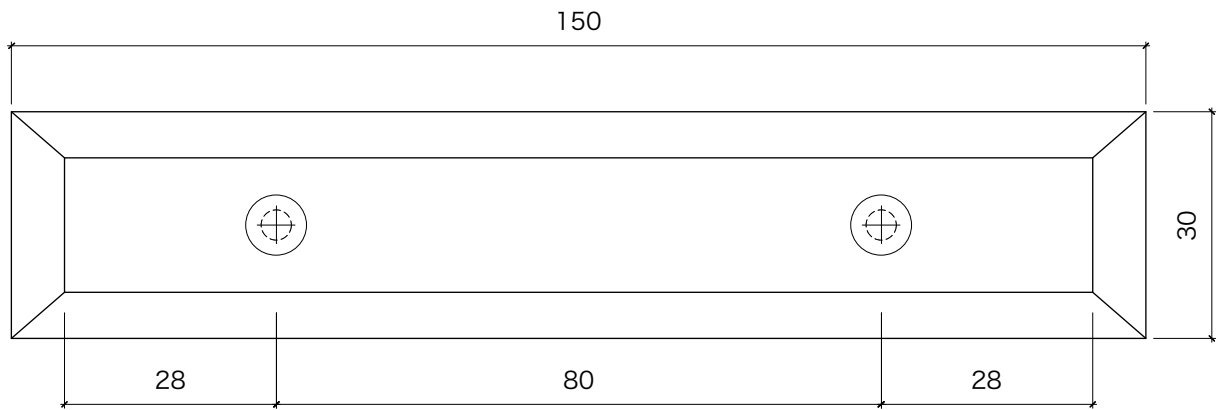
背面図
