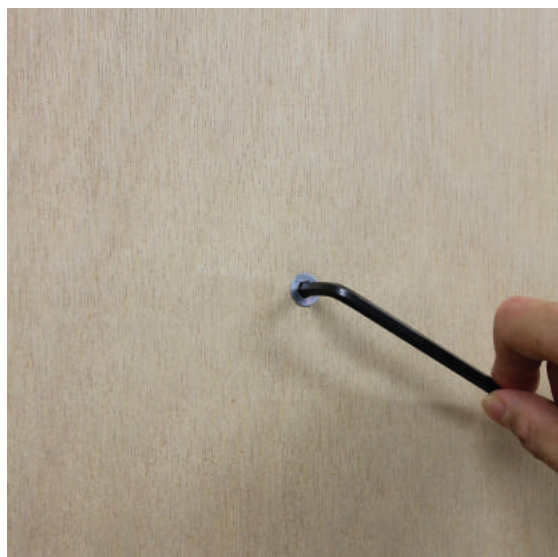
04_ 六角レンチで鬼目ナットを回して、ねじ込んでいきます。設置面の表面まで埋まったら止めます。
