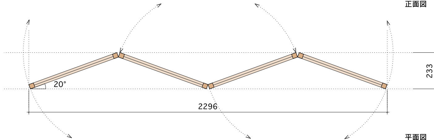
正面図
