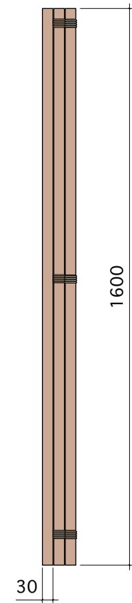
断面図
