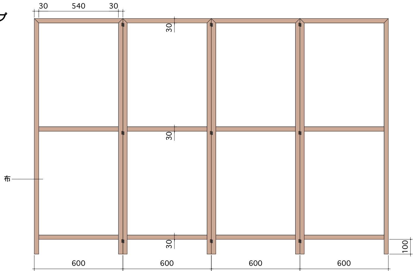
正面図
