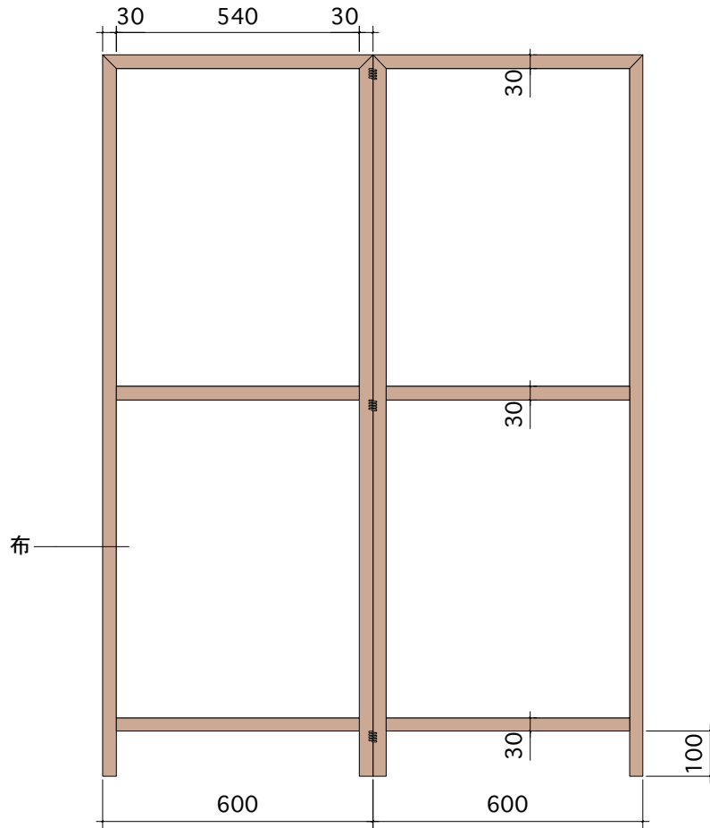
正面図
