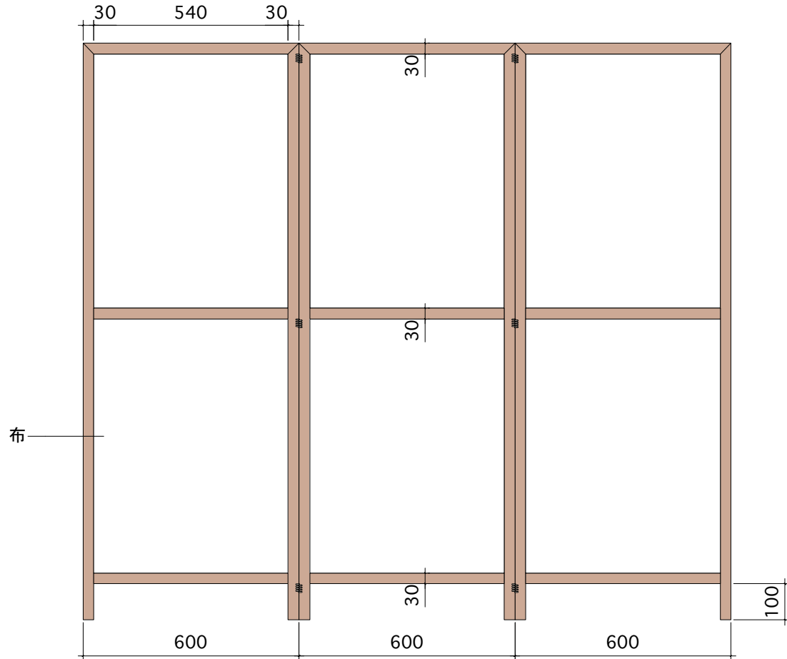
正面図
