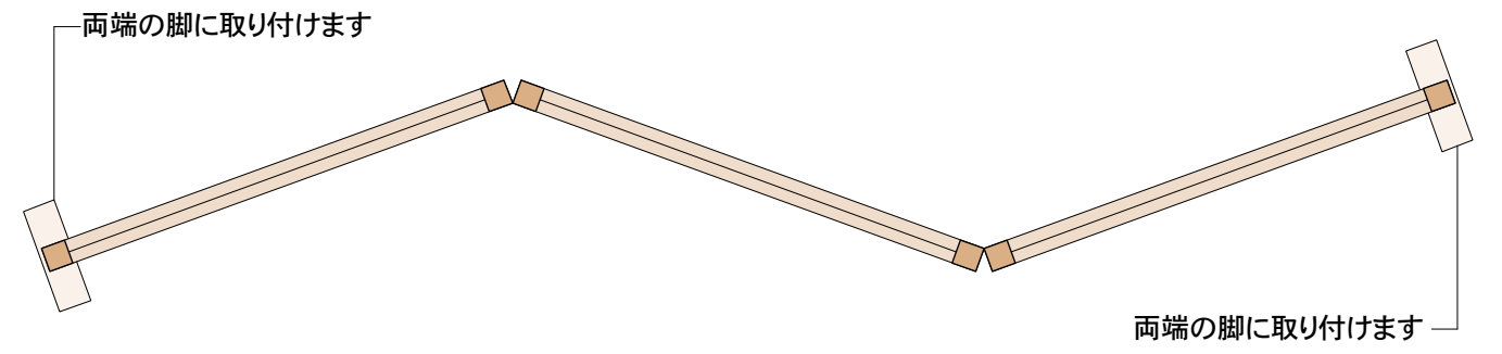
平面図 S=1/10
